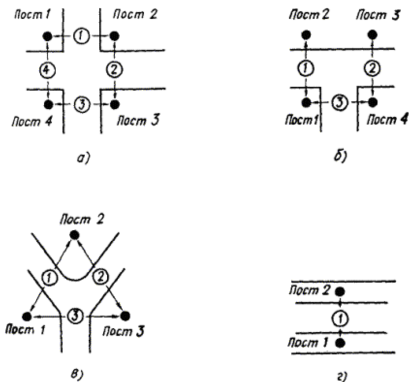
Рис. 1. Схема расстановки постов для подсчета интенсивности пешеходного движения
