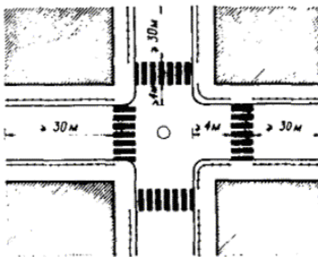
Рис. 6. Установка направляющих пешеходных ограждений на регулируемом перекрестке
