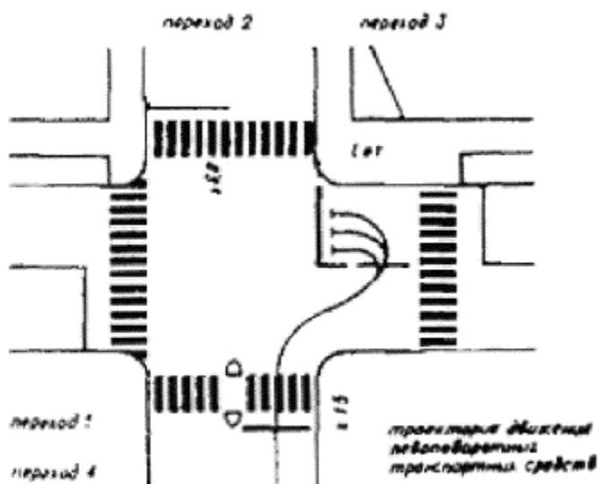
Рис. 3. Расположение наземных пешеходных переходов в зоне перекрестка
