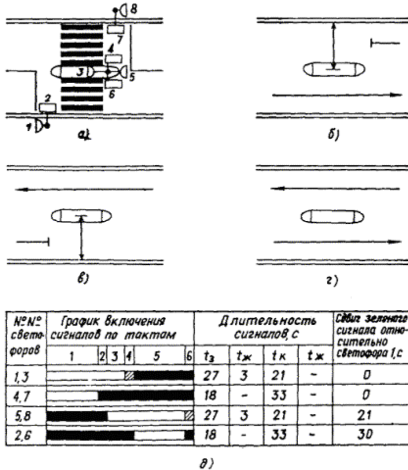
Рис. 10. Режим работы светофорной сигнализации на пешеходном переходе:
