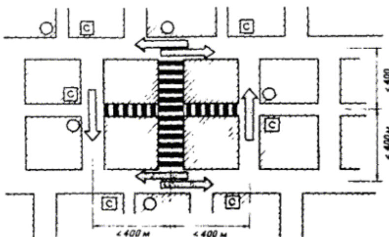
Рис. 7. Схема организации пешеходной зоны
