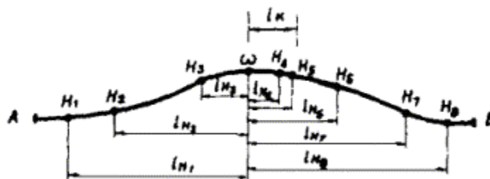
Рис. 2. Расчетная схема определения местоположения пешеходного перехода
