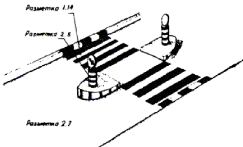
Рис. 5. Разметка пешеходного перехода
